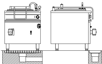
Рис. 4: Исполнение решетки с трапом
