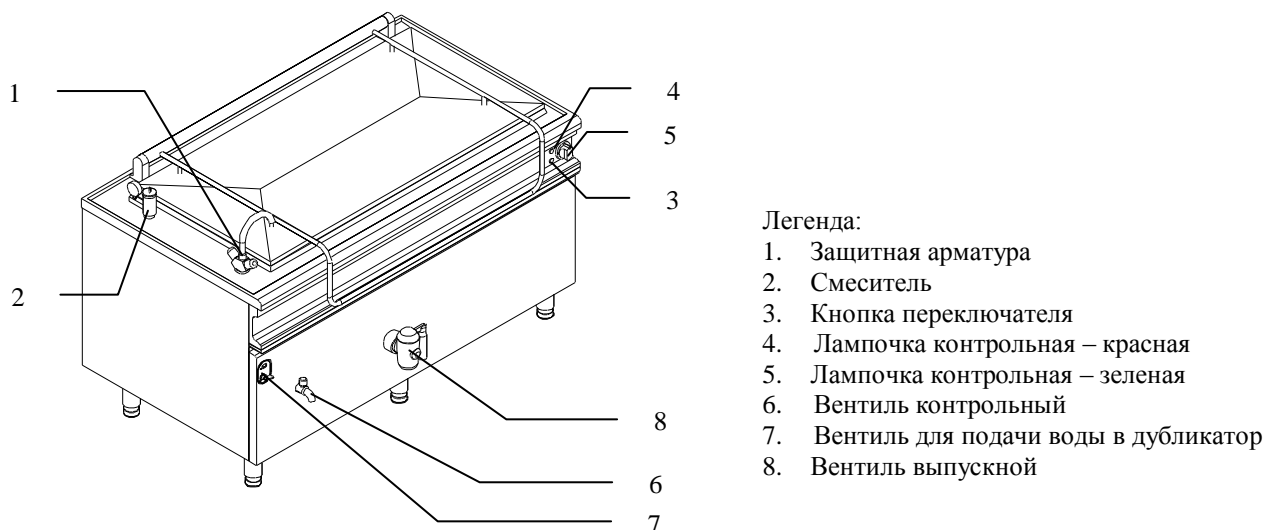
Рис. 1: Электрочотел
