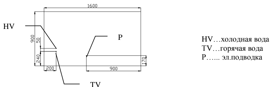
Рис. 3: Положения электроприсоединений на приборе
