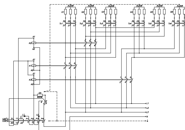
Рис. 2:Схема электросоединений
